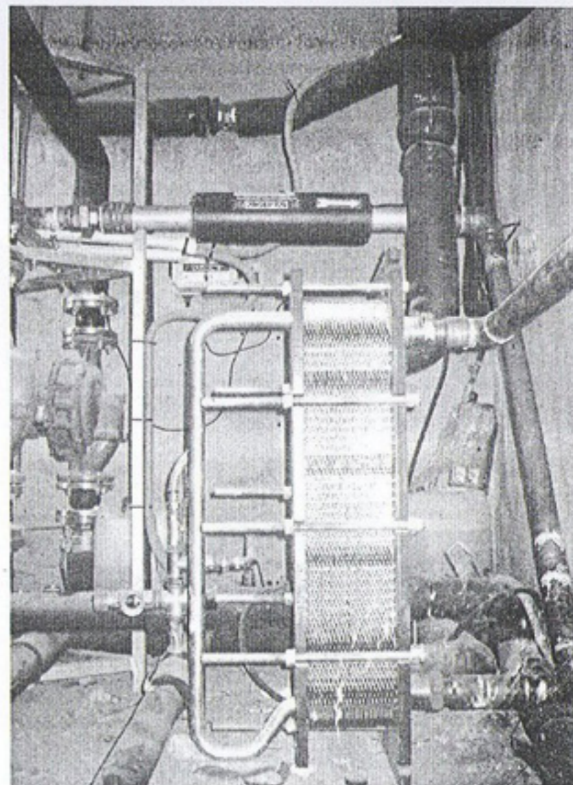
Sistema AQUASONIC instalado en el circuito de placas solares para el agua caliente
